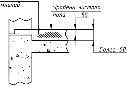
Вид Е
