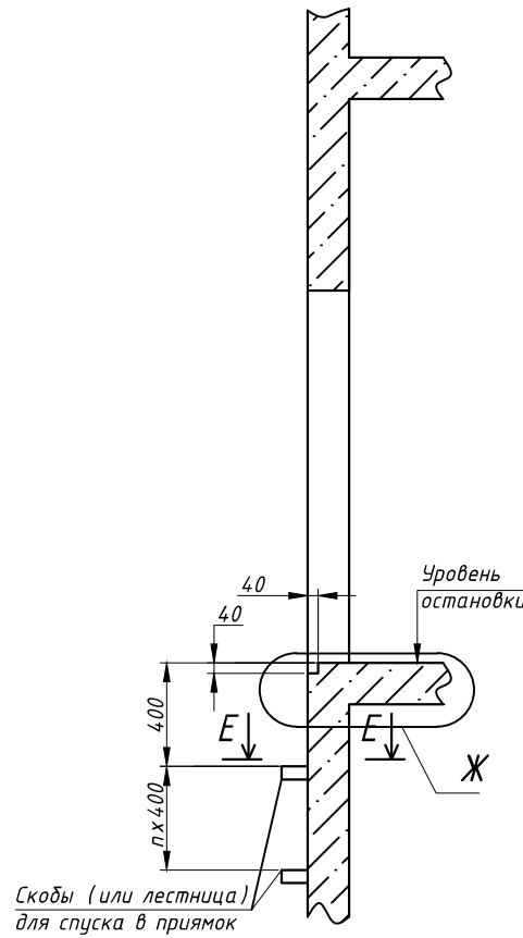
Вид Г
