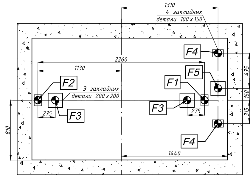
Направляющая противовеса
