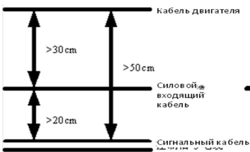
Рис2.(а)Параллельная прокладка
