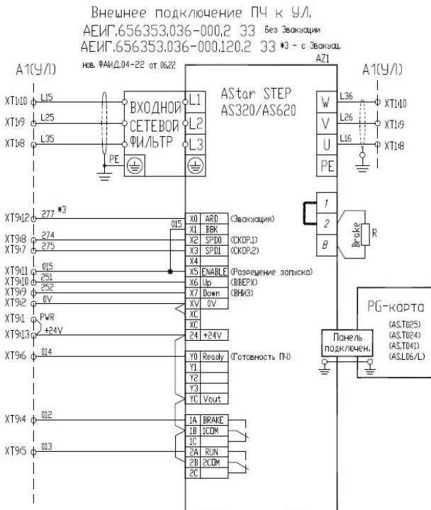
Рис. 3г Подключение ПЧ AS 620/AS320 к станции УЛ с установкой вне шкафа.
