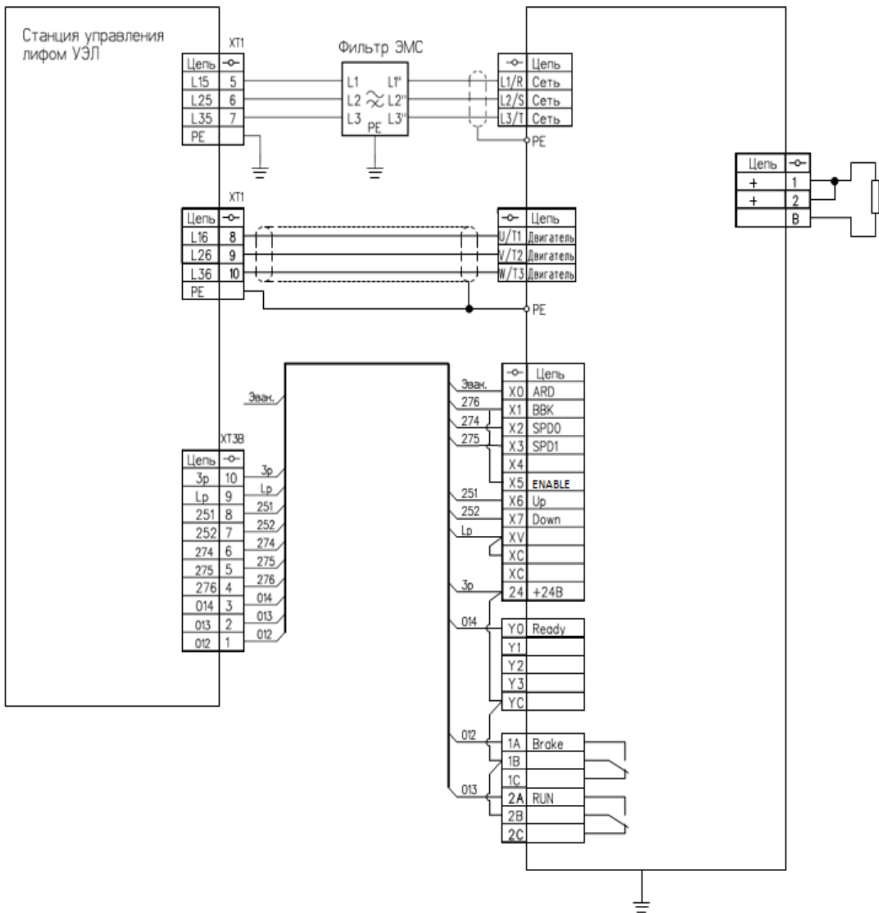
Рис. 36 Подключение ПЧ AS 620/AS320 к станции УЭЛ
