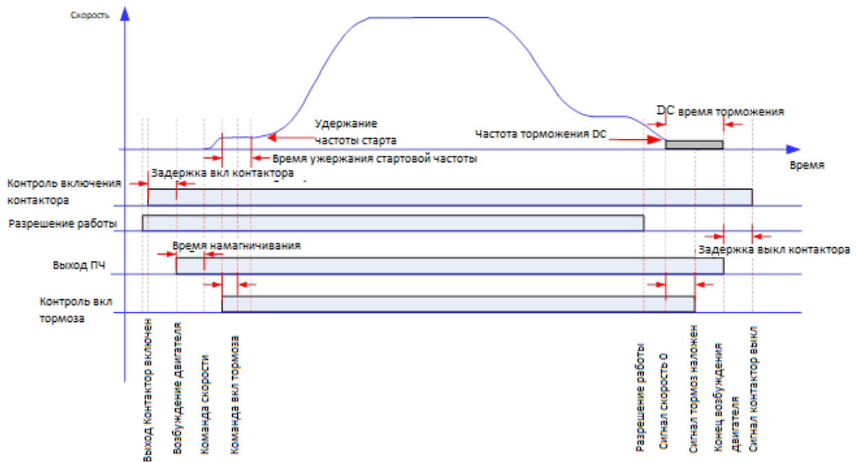
Рис.12 Алгоритм работы ПЧ без энкодера
