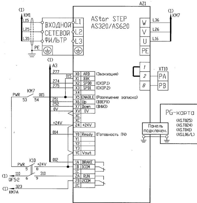
Рис. 3в Подключение ПЧ AS 620/AS320 к станции УЛ со встроенным ПЧ в шкаф
