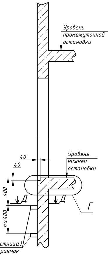
Вид Б
