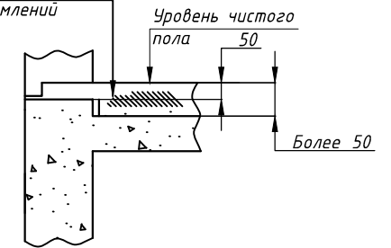
Вид Ж (вар.2) (подливка чистого пола более 50 мм.)
