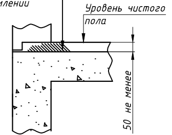
Вид Ж (вар.2) (подливка чистого пола более 50 мм.)
