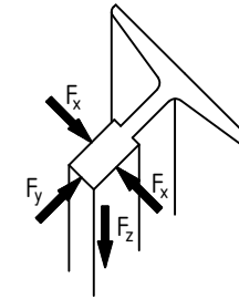
Направляющая противовеса
