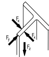
Направляющая противовеса
