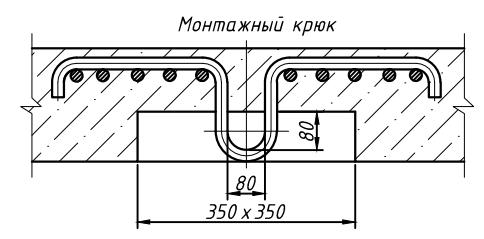
Вид Е
