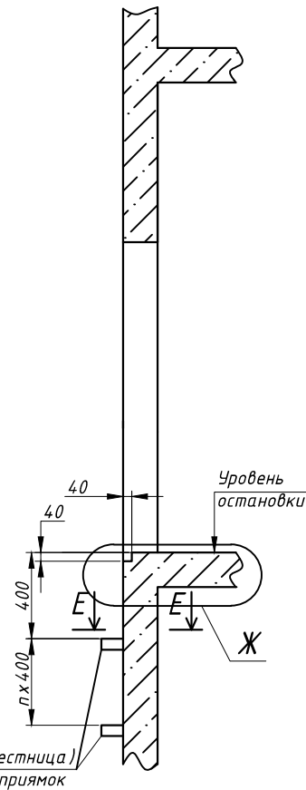
Вид Г
