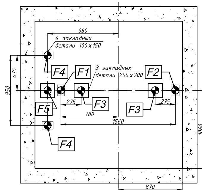
Направляющая противовеса
