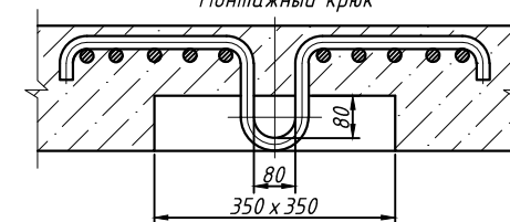
Вид Е
