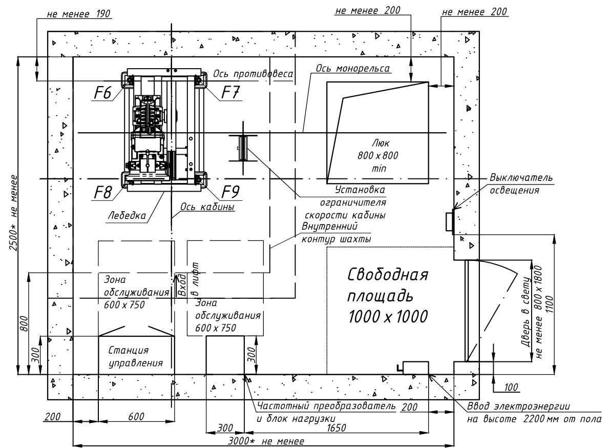
А-А Машинное помещение (примерное расположение)
