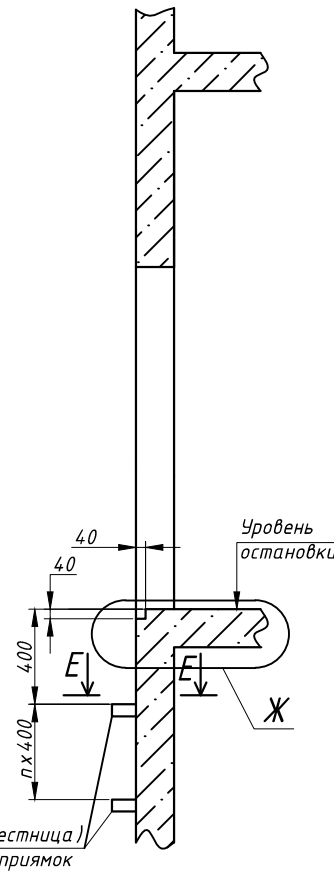
Вид Г
