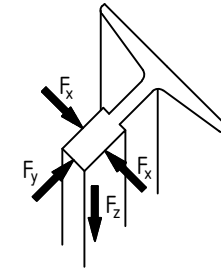
Направляющая противовеса
