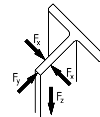
Направляющая противовеса
