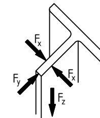
Направляющая противовеса
