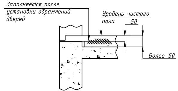
Вид Ж (вар.2) (подливка чистого пола более 50 мм.)
