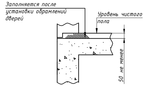
Вид Ж (вар.2) (подливка чистого пола более 50 мм.)
